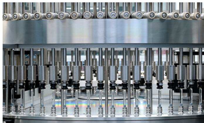
Ligne de remplissage de cartouches injectables
